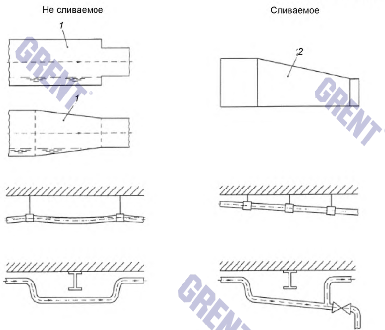
Рисунок А.13 – Дренаживание трубопроводов
