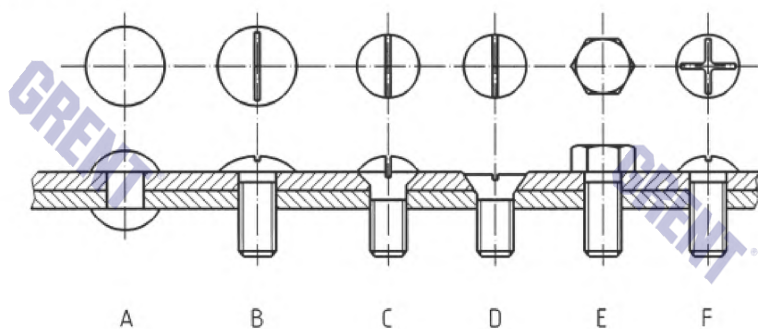
Рисунок А.22 – Крепежные изделия для зоны разбрызгивания
