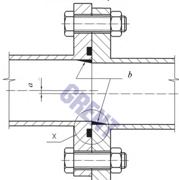
Рисунок А.5 — Неразъемные соединения. Сварные трубы
